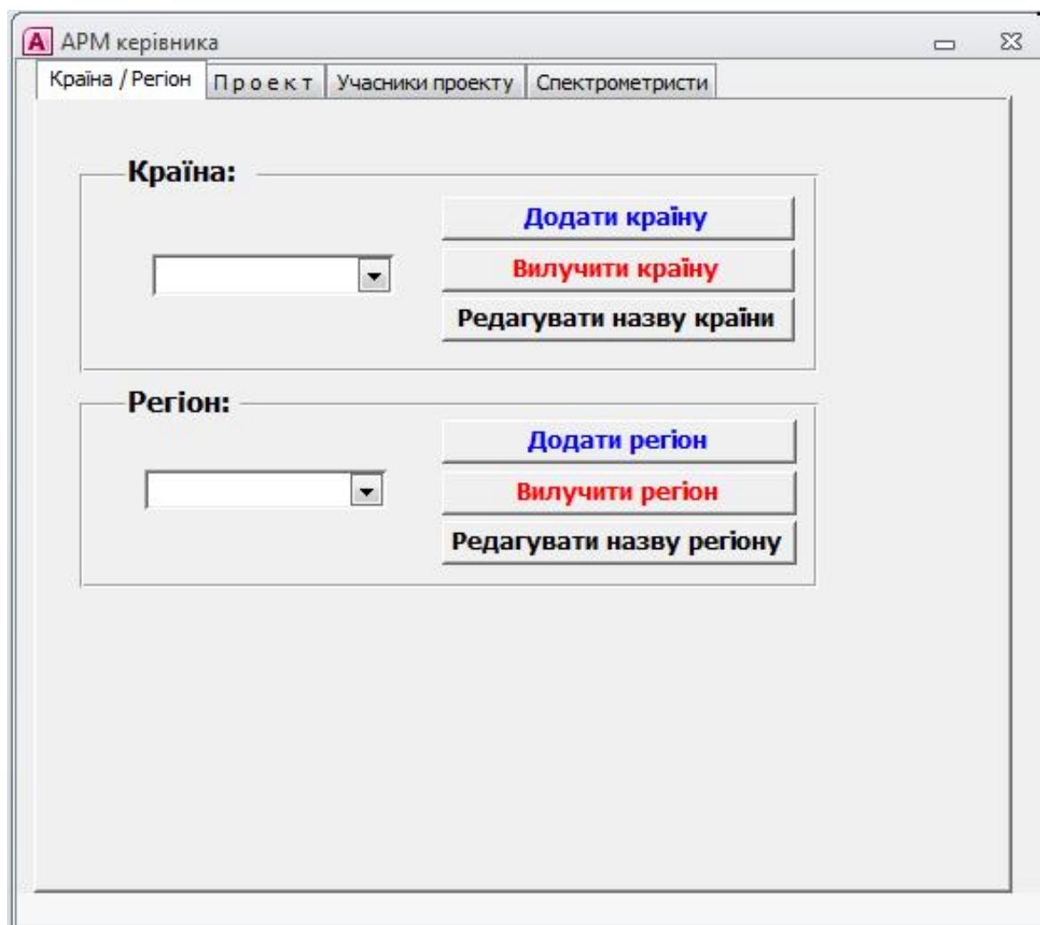
Рис. 2. Операционные вкладки АРМ “Руководитель”
