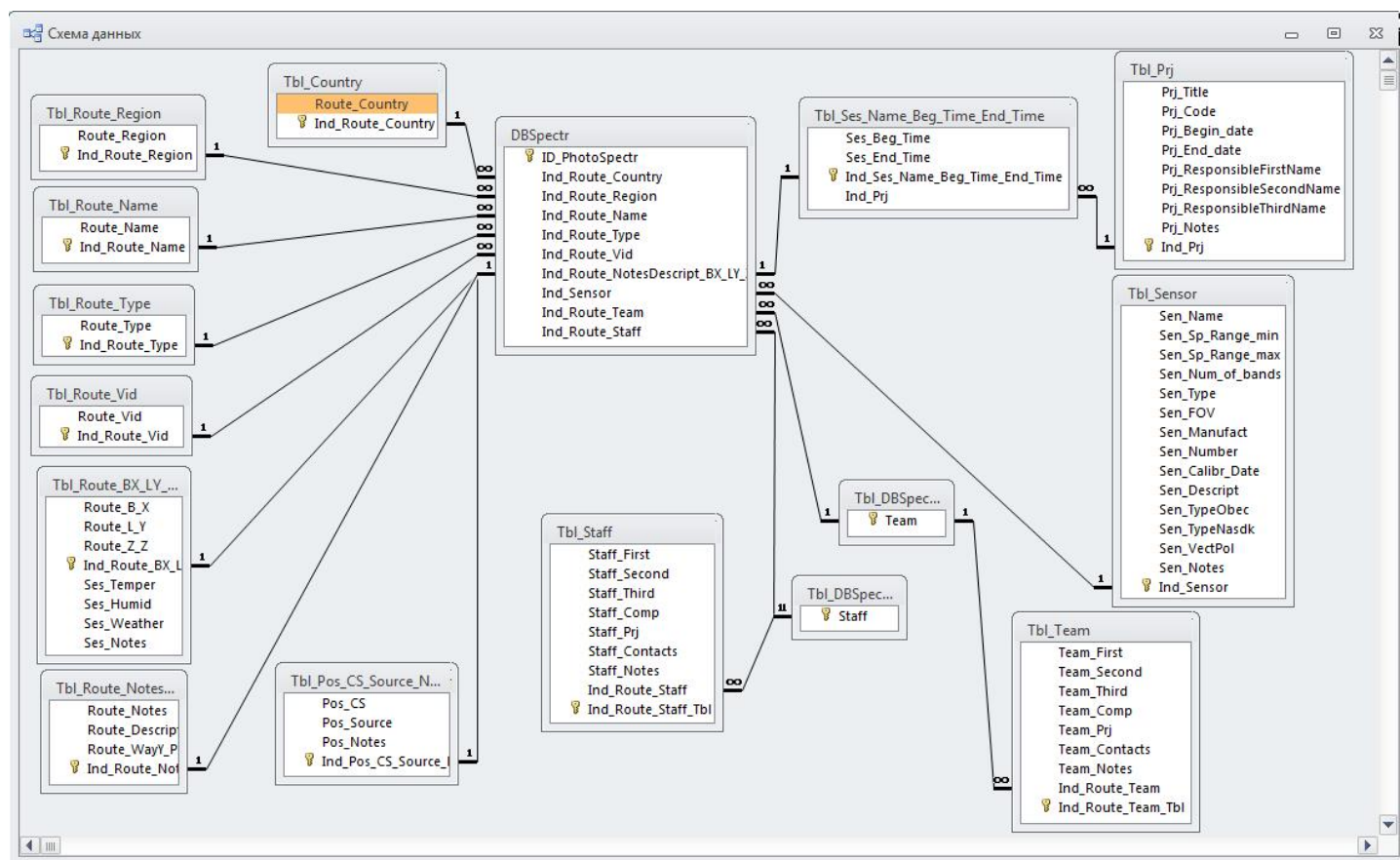
Рис. 1. Схема БД на основе реляционной модели
