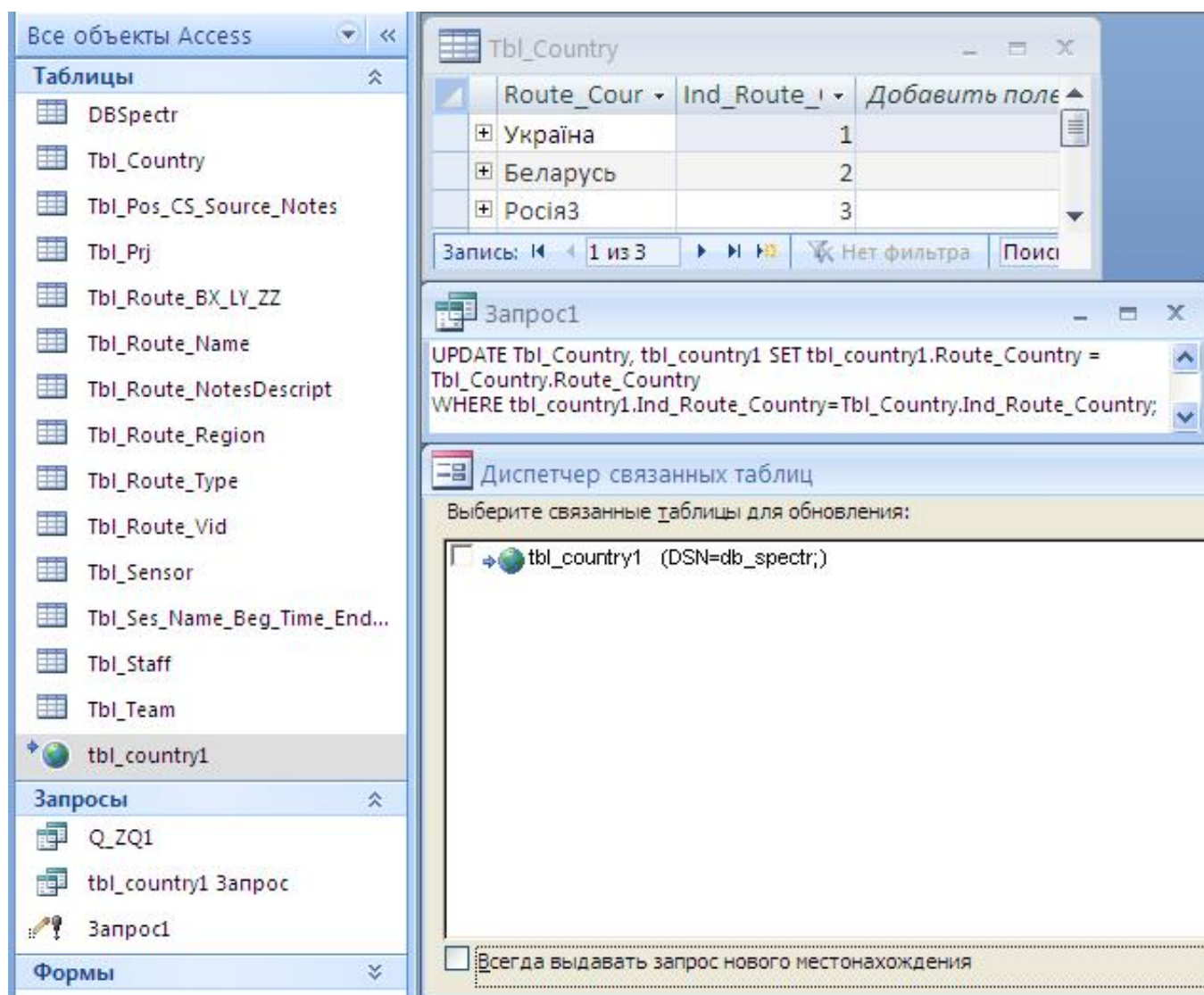
Рис. 11. Вид SQL-запроса синхронизации БД Access и MySQL
