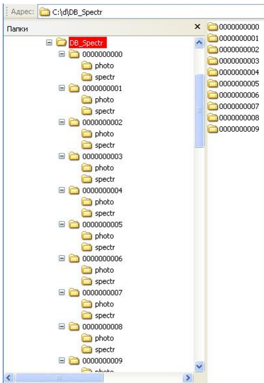
Рис. 6. Система каталогов спектральных данных и их атрибутов
